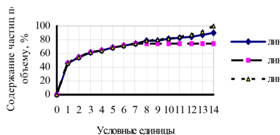
Рис. 4. Принятое содержание частиц по объему для различных смесей
