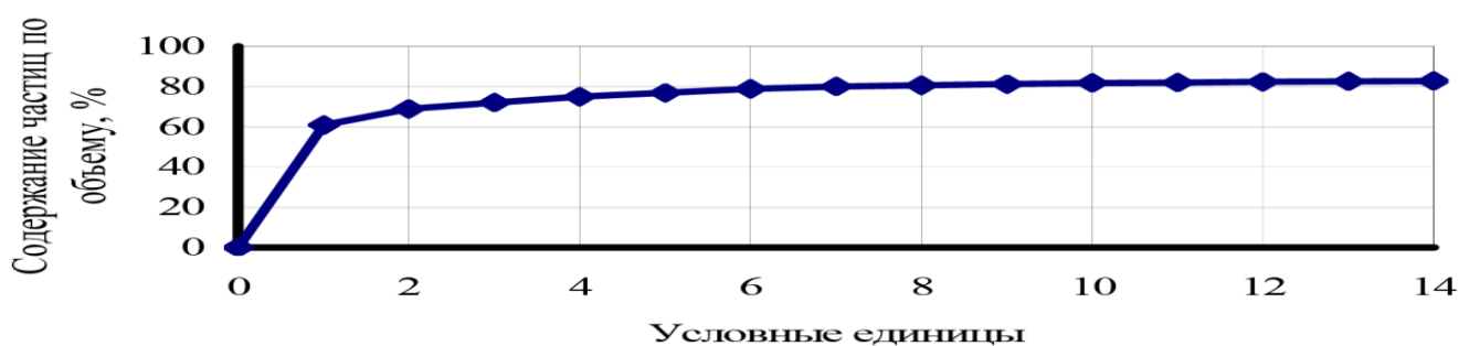
Рис. 2. Результаты расчета предельной теоретической кривой; условные единицы соответствуют диаметрам отверстий сит, указанных в табл. 1.
