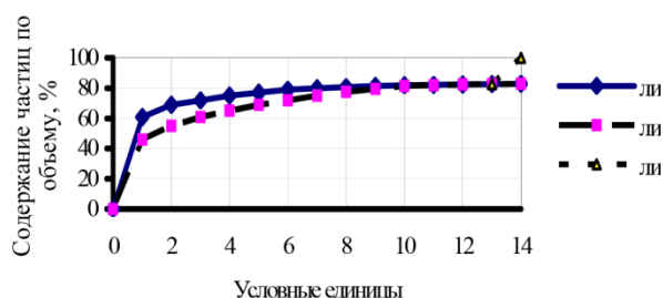
Рис. 3. Предельная теоретическая и принятая предельная фактическая кривые
